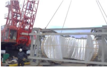
《起重機船※6を使用する荷役作業》
